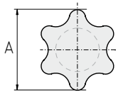
CALIBRO DI CONTROLLO PER IMPRONTA TORX CHECK GAUGE FOR TORX MARK
